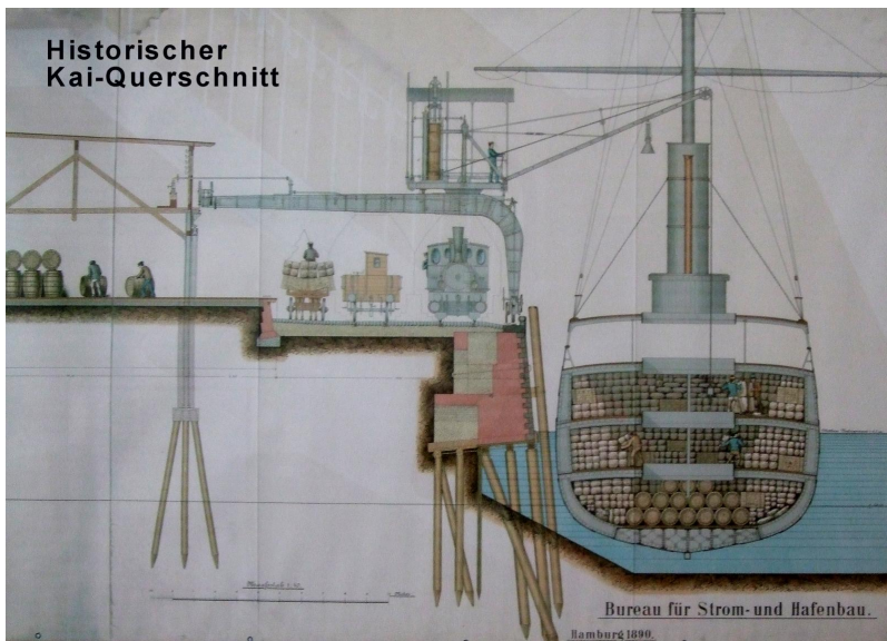
Historischer prinzipieller Kaiquerschnitt
