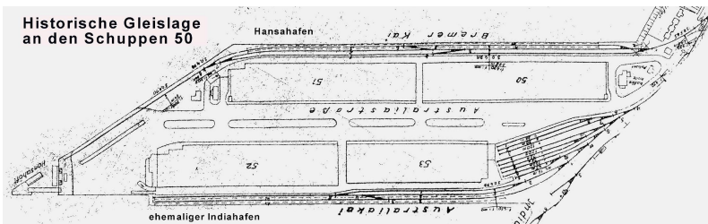
Gleislage 2004 am Bremer Kai
